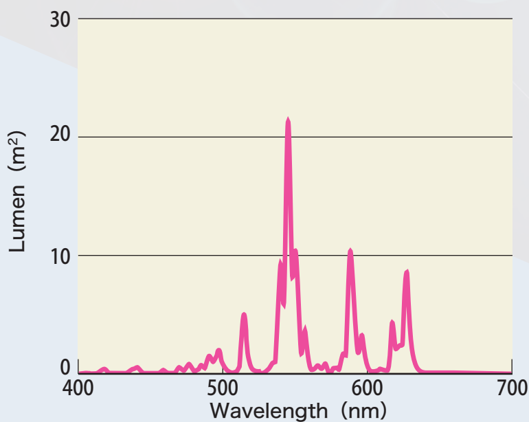
励起、発光スペクトル Excitation emission spectra
