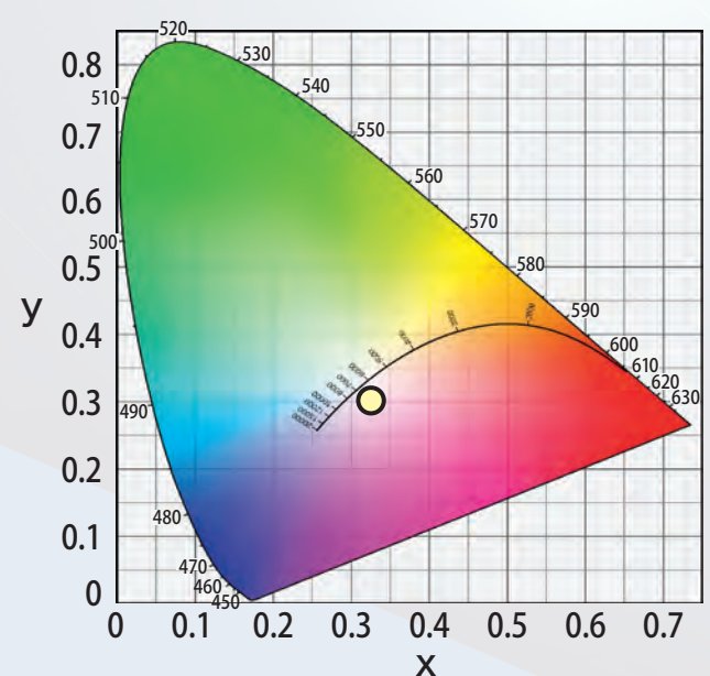
発光色度図 Chromaticity diagram
