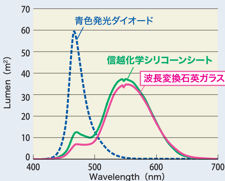
励起、発光スペクトル Excitation emission spectra
